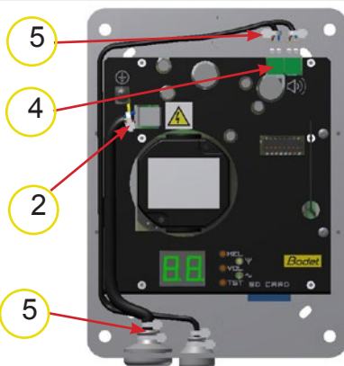
Précaution d'installation des Melodys TBT 24V : distance maximale à respecter
