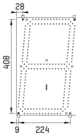
Módulo LED de 42 cm
