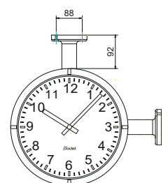
Doppelseitiger Träger
