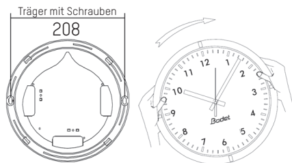
Einseitiger Wandträger
