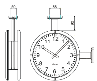
Doppelseitiger Träger
