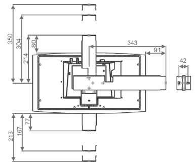
Opalys 14 auf einem doppelseitigen Halter
